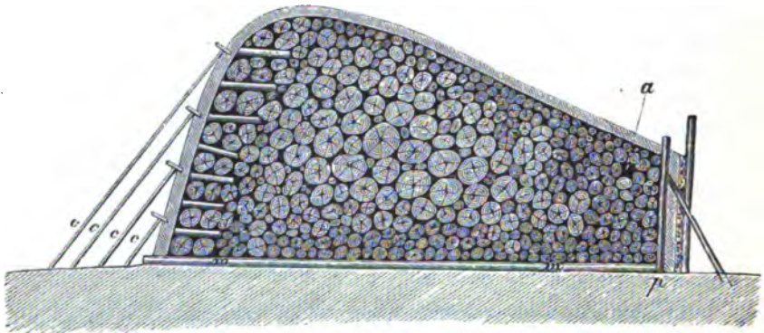
Fig. 317.—Horizontal kiln.
